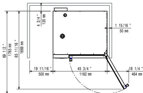
Felülnézet
